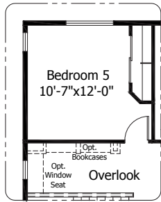
Optional Bedroom 5
